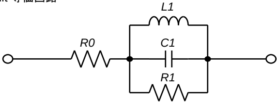
Part Number 品番 Equivalent Circuit Parameters 等価回路パラメータ R0 (mΩ) L1 (μH) C1 (pF) R1 (kΩ)
