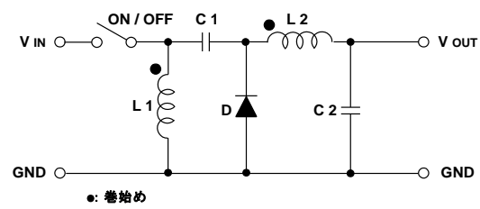
【ZETA Converter】
