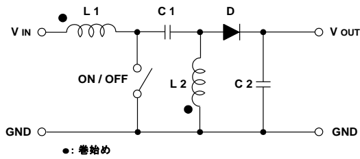
【SEPIC Converter】
