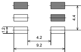
Recommended Land Pattern 推奨ランドパターン
